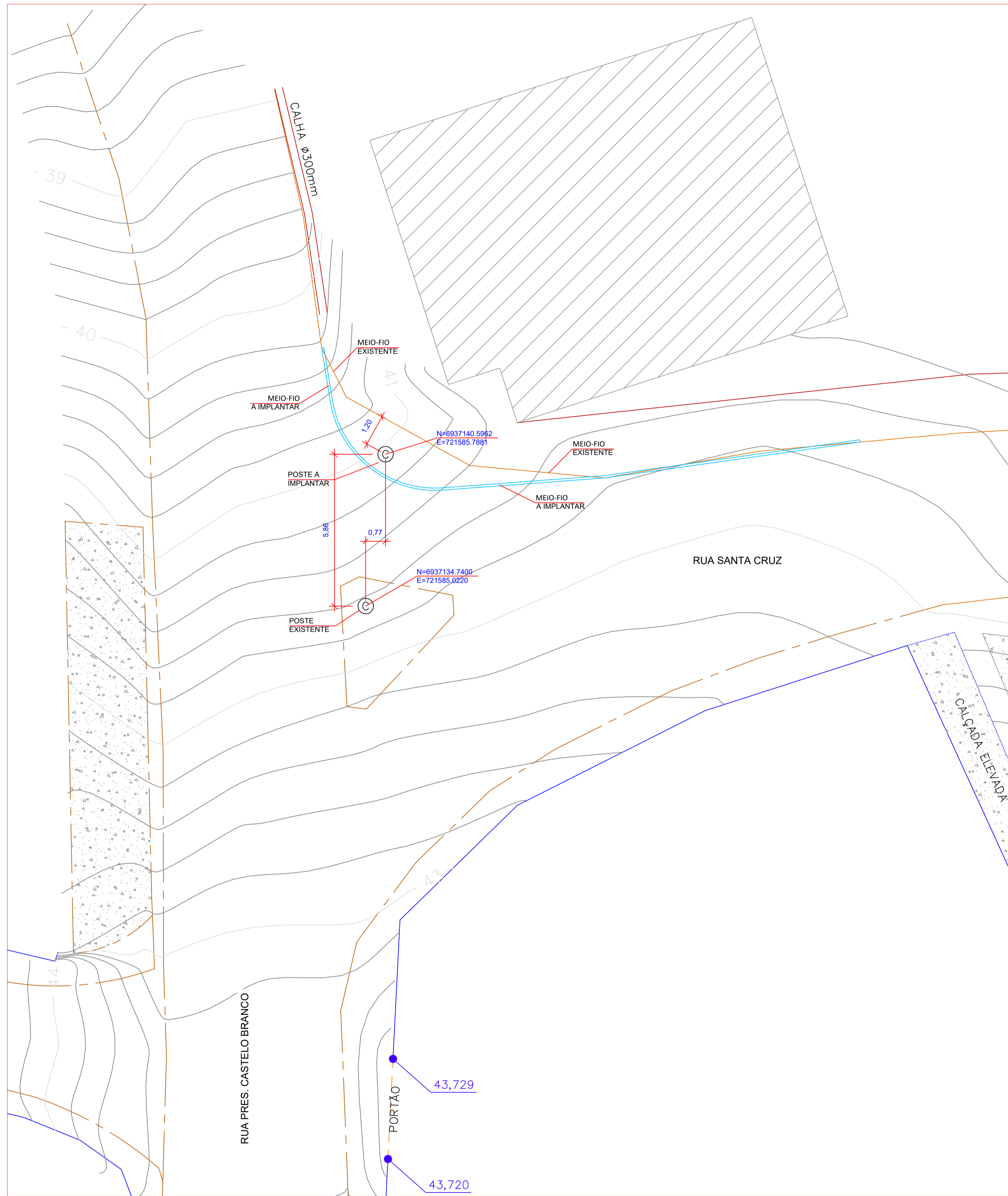
1 LOCAÇÃO - REALOCAMENTO DO POSTE ESCALA 1:100
