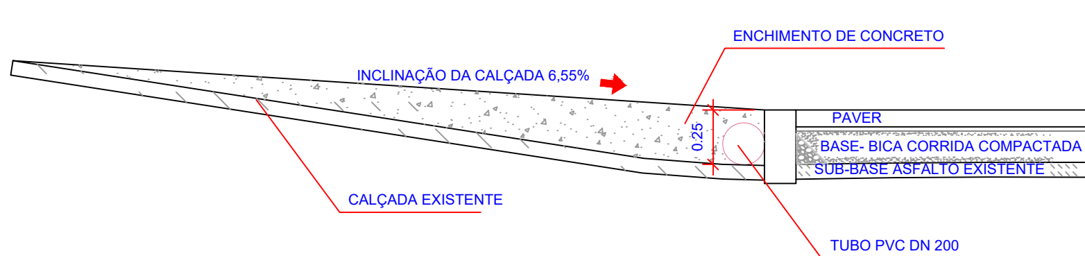
3) SEÇÃO BB ESCALA 1:20
