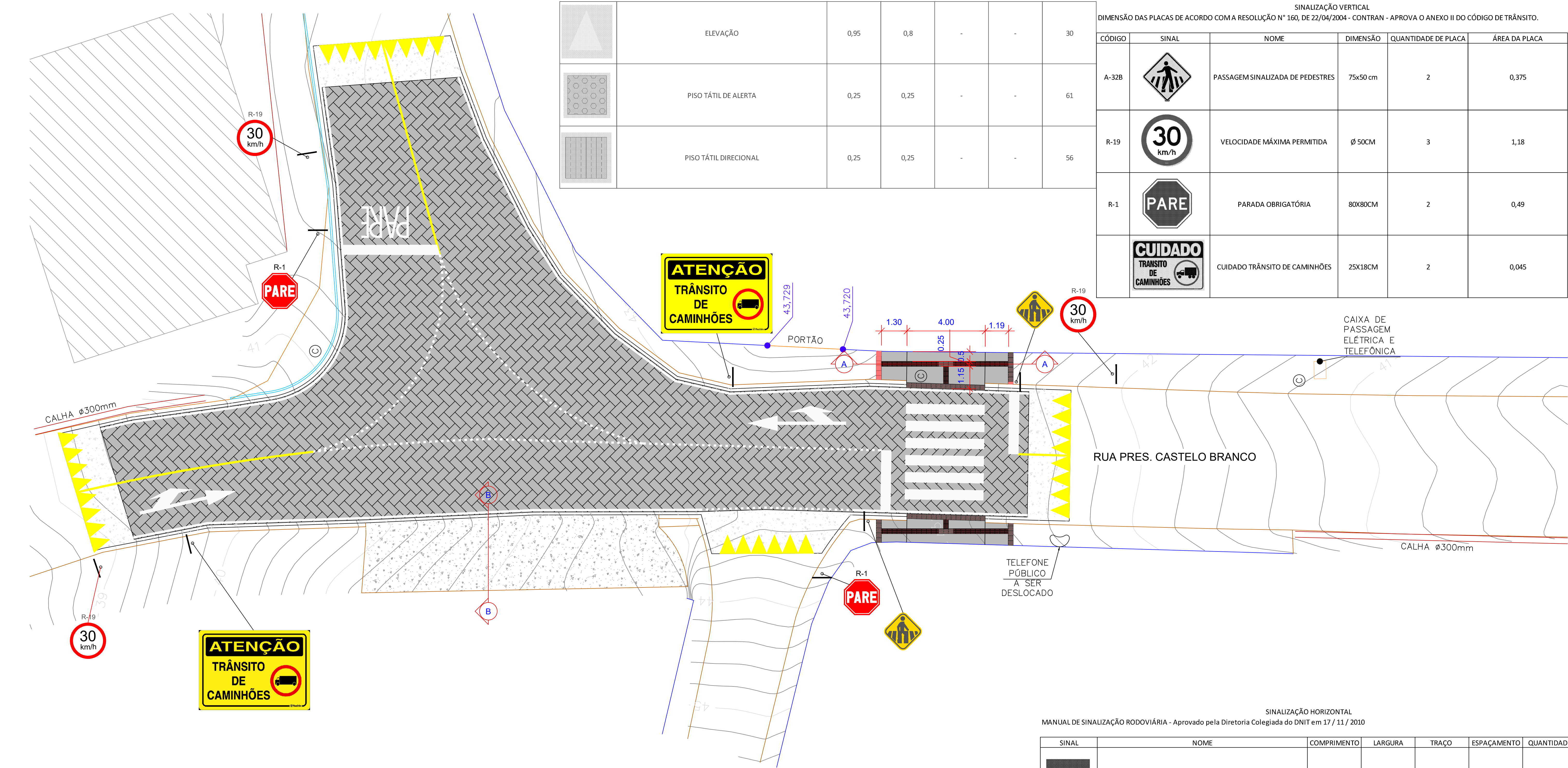
1) LOCAÇÃO DAS SINALIZAÇÕES HORIZONTAIS/VERTICAIS ESCALA 1:200
