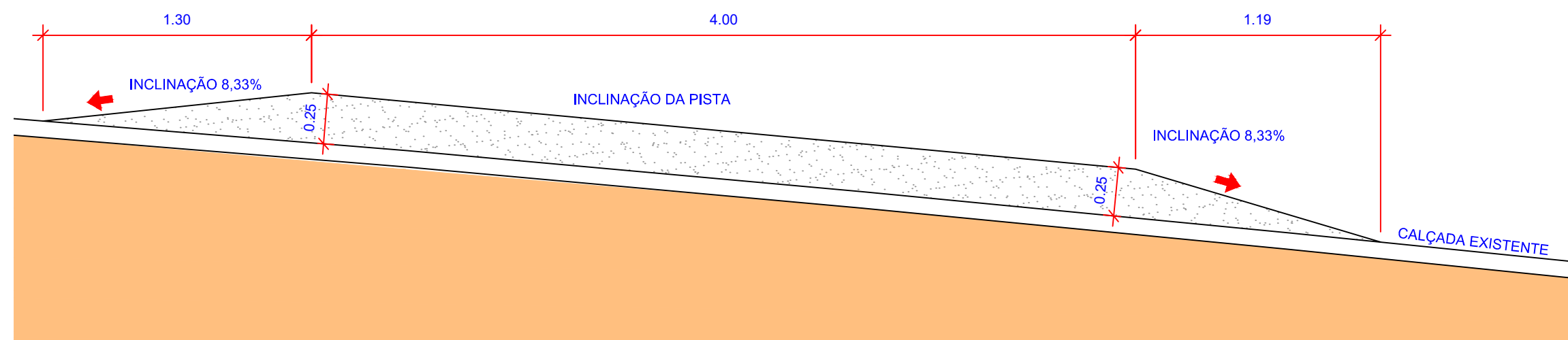
2) SEÇÃO AA ESCALA 1:20
