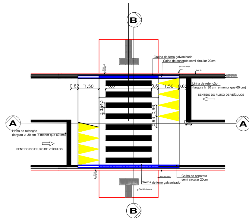
PASSEIO ELEVADO NA VIA (GENÉRICO)
