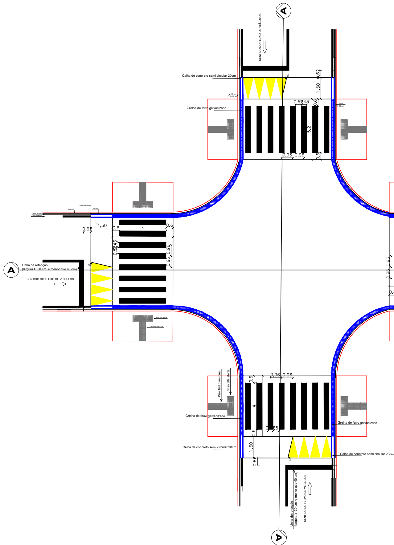
PASSEIO ELEVADO NO CRUZAMENTO (GENÉRICO )
